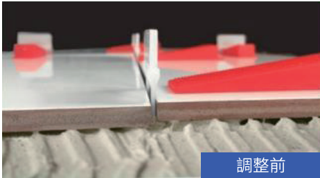
使用前:目地部で段差が発生する。
