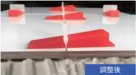
使用后:目地部の不陸が無くなる。
