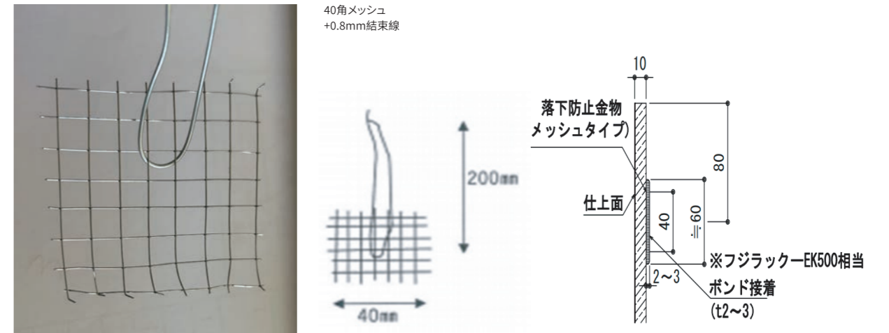
落下防止付金物メッシュタイプ
